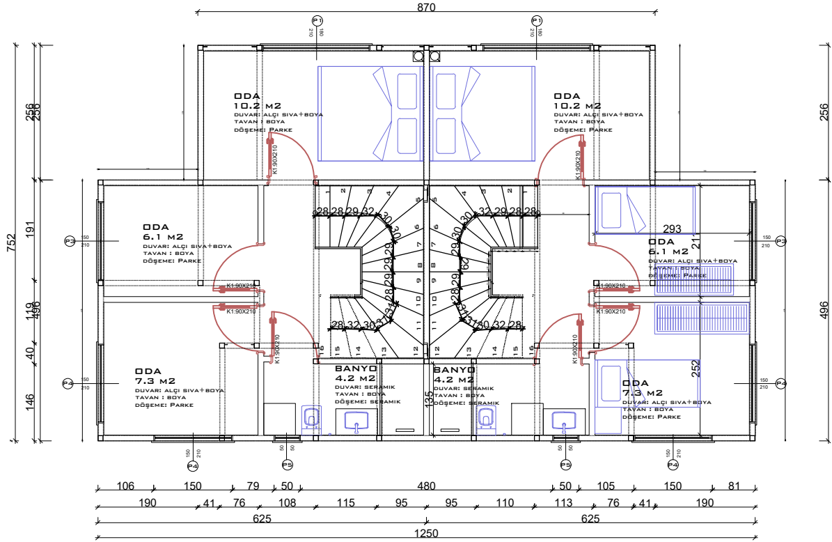
A VE B BLOK 1. KAT
