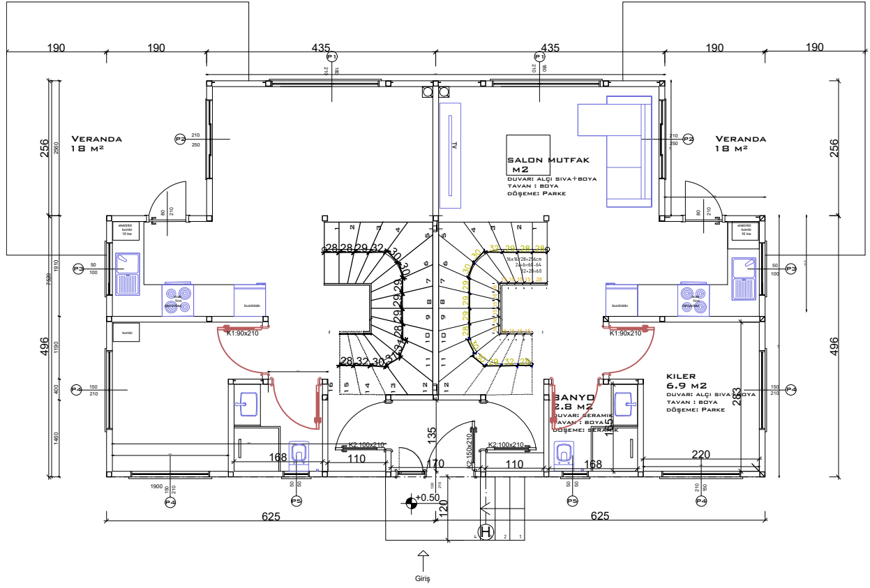
A VE B BLOK ZEMİN KAT
