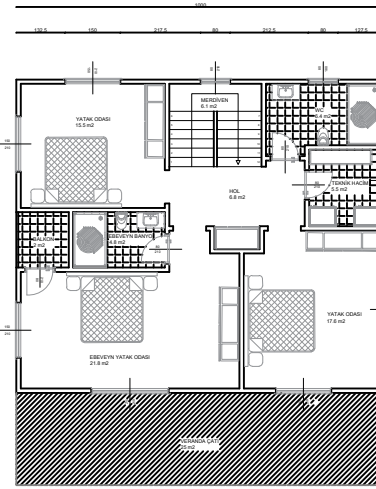
1. KAT 82 m²
